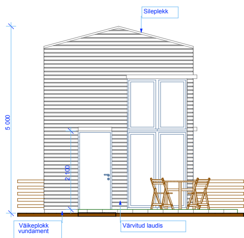
1 VAADE EEST 1:100
