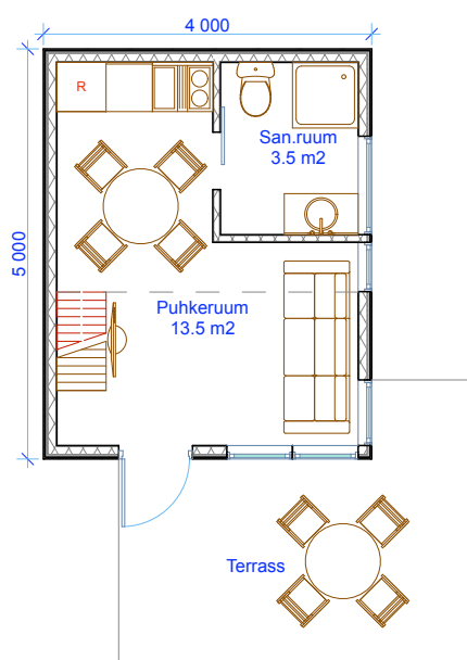
3 I KORRUSE PLAAN 1:100
