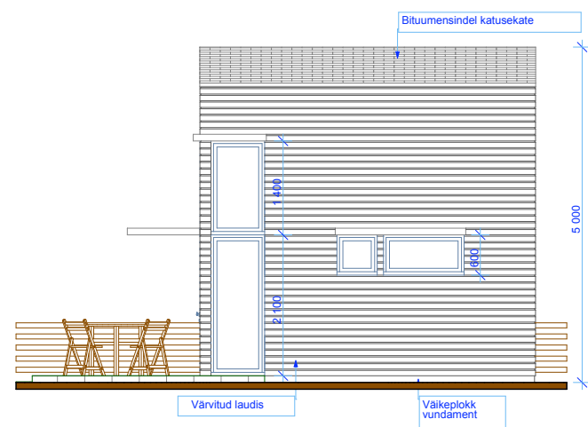
2 VAADE PAREMALT 1:100
